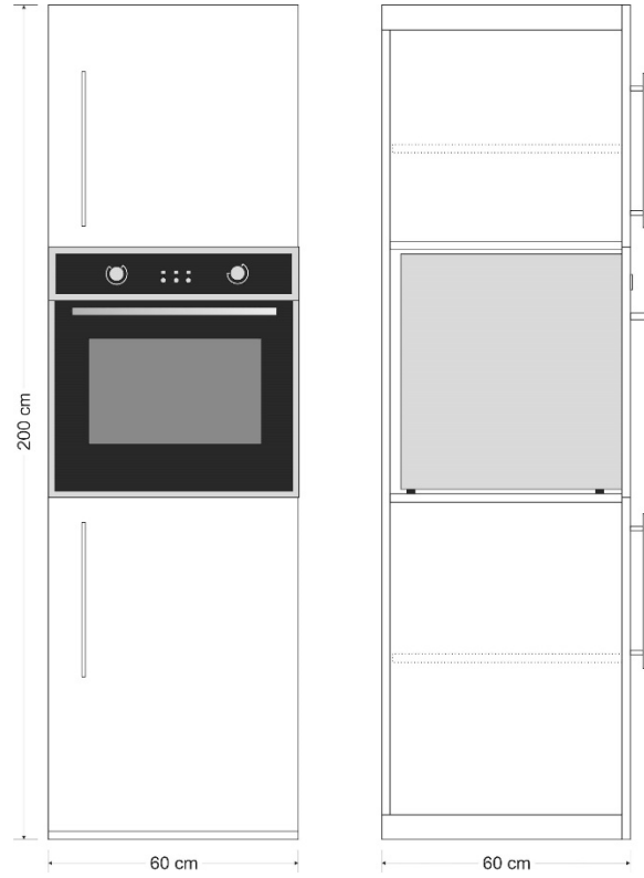
Höhe 200 cm mit Backofen
